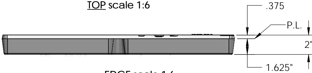
EDGE scale 1:6
